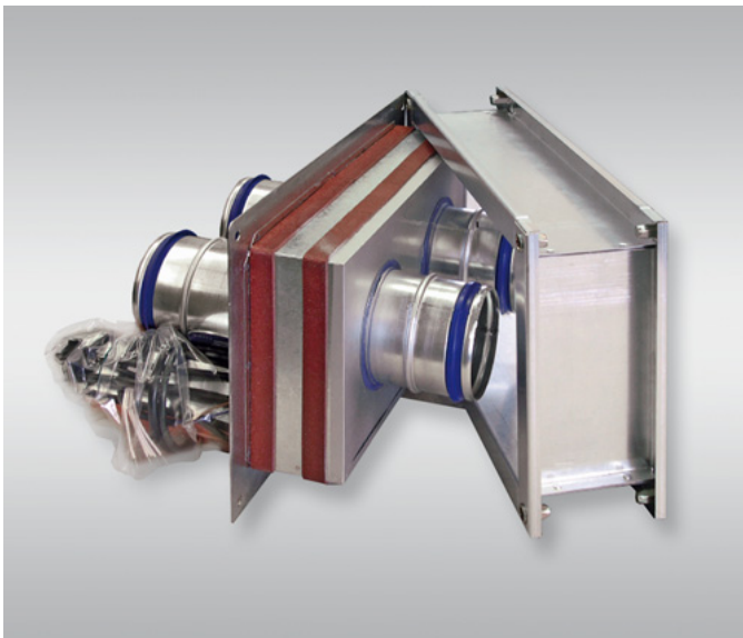
Objektspezifische Sonderlösung: Brandschutzklappe FKRS in Zwillingsausführung Customised special solution: Fire damper FKRS in side by side installation
